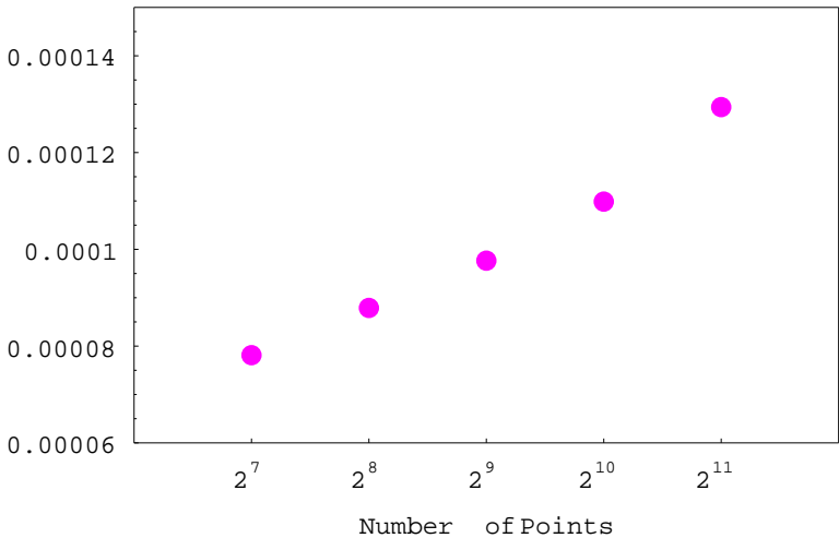
CPU Time per Point
