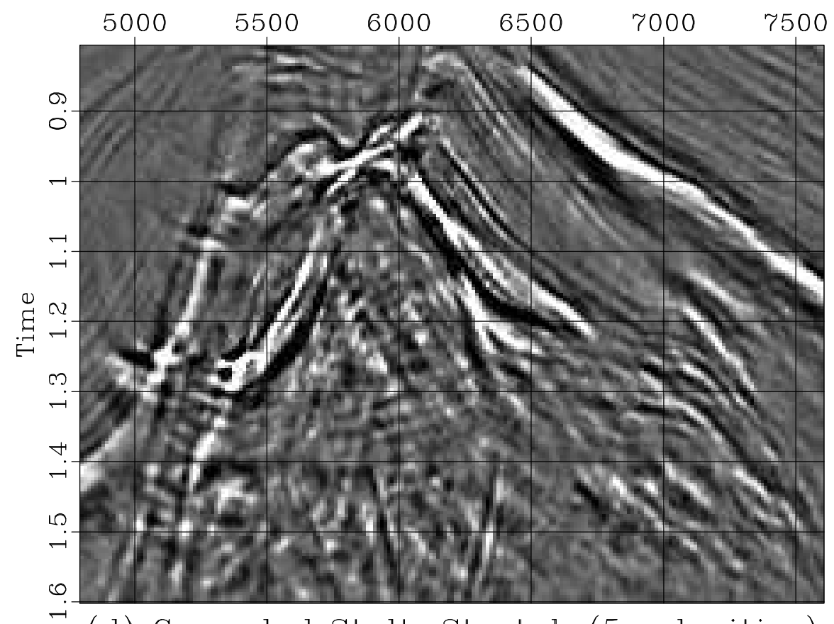
(d) Cascaded Stolt-Stretch (5 velocities)
