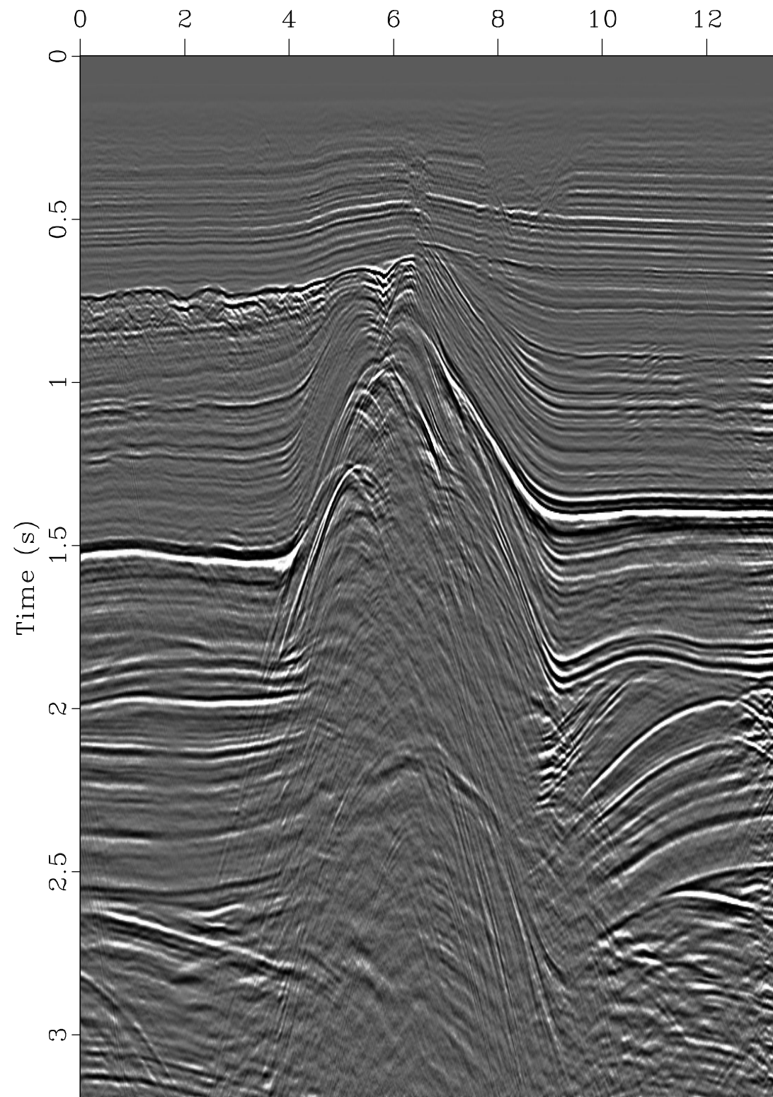
NMO Stack
